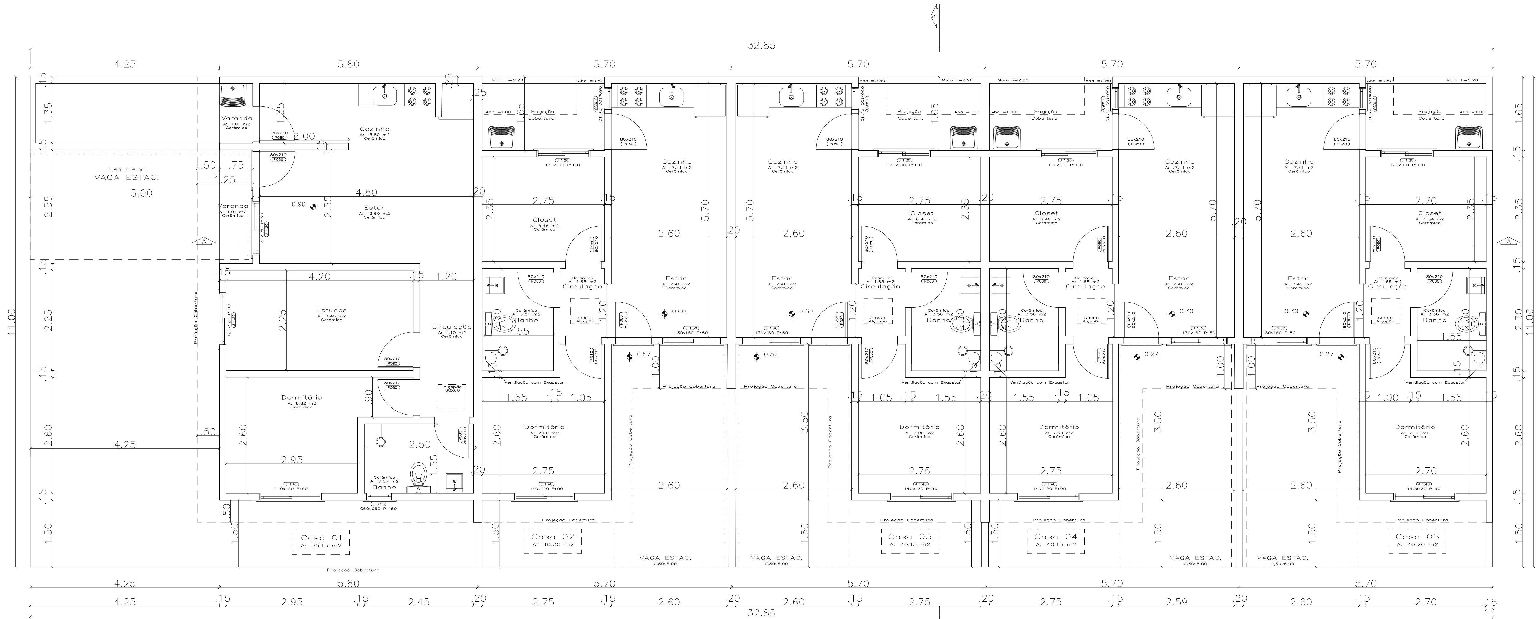
PLANTA BAIXA 215,95m²
